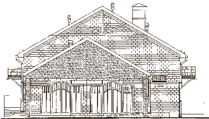
ELEWACJA PÓŁNOCNA
