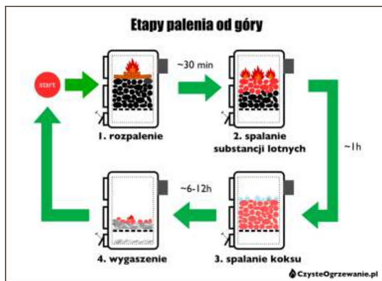
Palenie rozpoczyna się od góry, dzięki czemu rozpoczęty zostaje proces dokładnego i oszczędnego spalania
